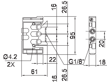
Simple piloto
