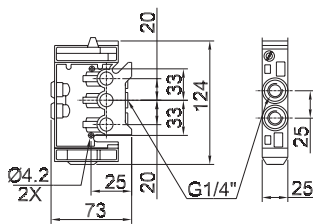
Válvula sem atuador
