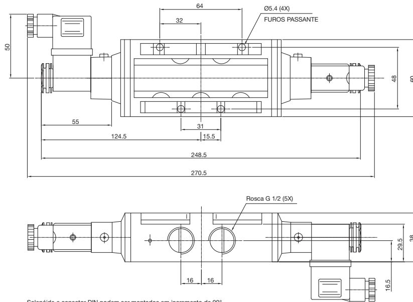
Solenóide e conector DIN podem ser montados em incremento de 90°
