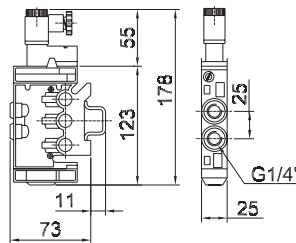
Simple solenóide
