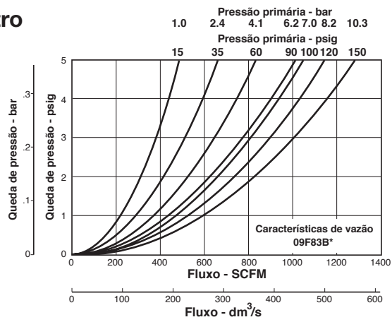
Regulador
