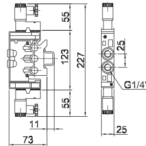
Duplo solenóide
