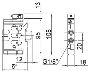
Simple piloto
