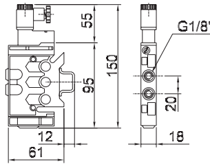
Simple solenóide
