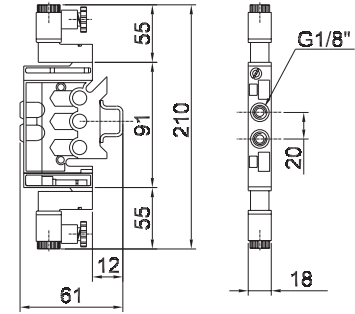
Duplo solenóide
